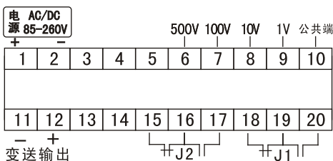
HB4740接线图
