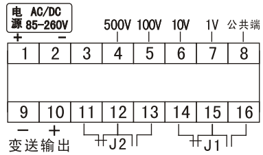
HB5740接线图
